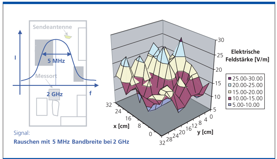
Bild 2. Feldstärkeverteilung in einer Ebene, gemessen unter Laborbedingungen.
