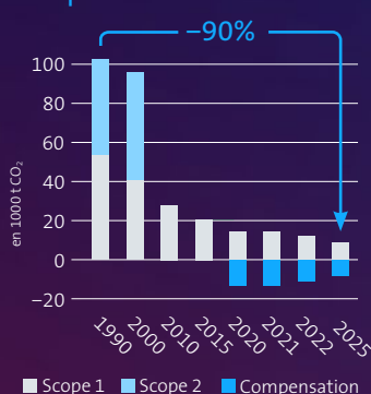
Scope 1 et 2
