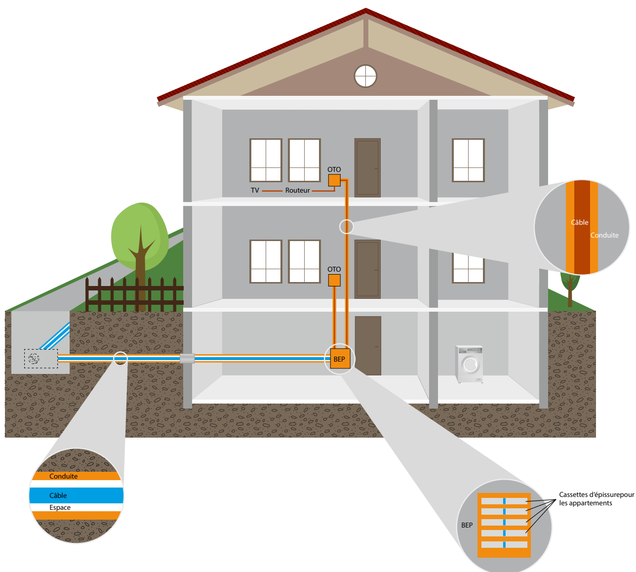
Figure 2: raccordement de communication – étapes et compétences pour les travaux à effectuer, cf. tableau 3
