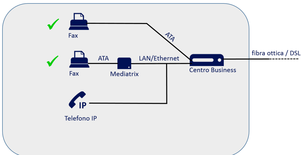
Figura 2: Smart Business Connect con impianto telefonico virtuale (hosted) e apparecchio fax analogico
