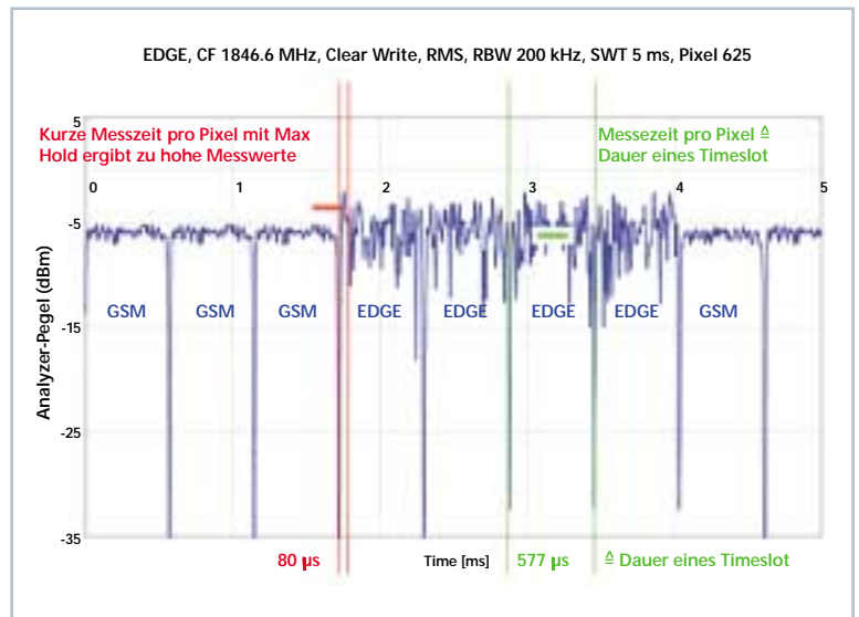
Bild 2. Bildung der RMS-Werte bei äquivalenten Timeslot-Leistungen GSM und EDGE (Darstellung zur Demonstration mit kleinerer Sweeptime als vorgeschlagen).
