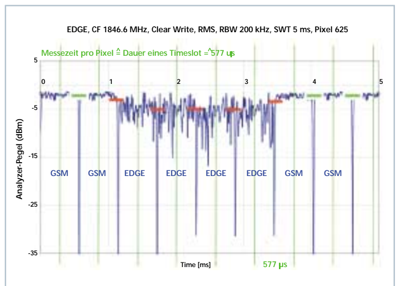
Bild 3. Bildung RMS-Werte bei reduzierten Timeslot-Leistungen von EDGE (Darstellung zur Demonstration mit kleinerer Sweeptime als vorgeschlagen).
