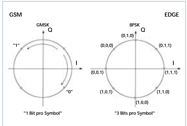
Bild 1. Modulation GSM und EDGE im IQ-Diagramm.
