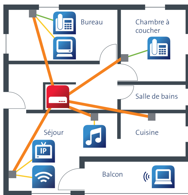
Ill. 17: câblage de réseau domestique structuré en étoile
