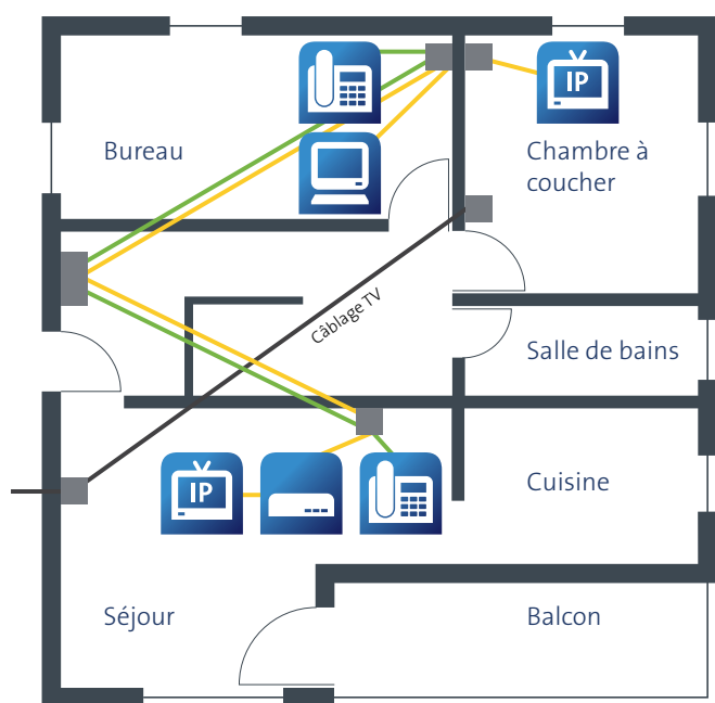
Ill. 16: aperçu de câblage de réseau domestique étendu
