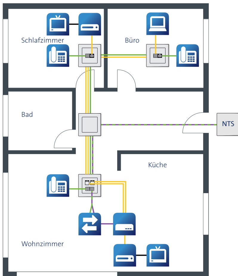
Abb. 7: Erweiterte Heimverkabelung Unterputz bei Kupferanschluss
