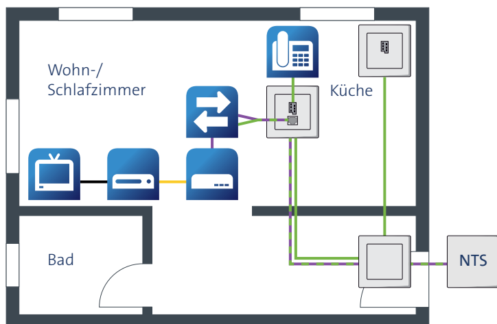
Abb. 4: Breitband-Internet-Hausinstallation
