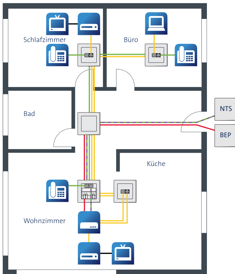
Abb. 8: Erweiterte Heimverkabelung Unterputz bei Glasfaseranschluss
