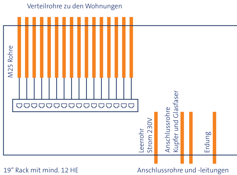
Abb. 13: Anschlussverteiler Mehrfamilienhaus
