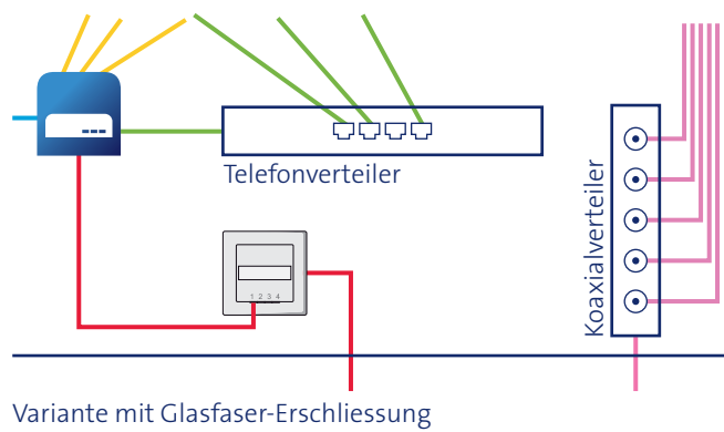
Abb. 10: Wohnungsverteiler mit Kabel-TV oder SAT-TV-Verkabelung
