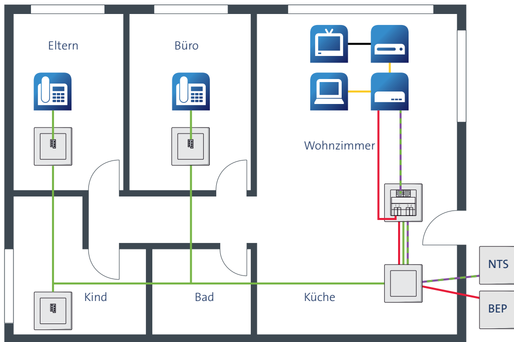
Abb. 6: Breitband-Internet-Hausinstallation (Glasfaser) ohne erweiterte Heimverkabelung
