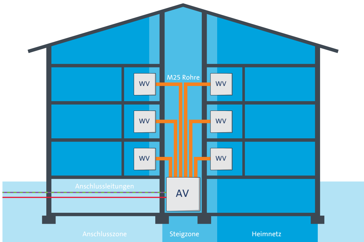
Abb. 12: Steigzone Mehrfamilienhaus
