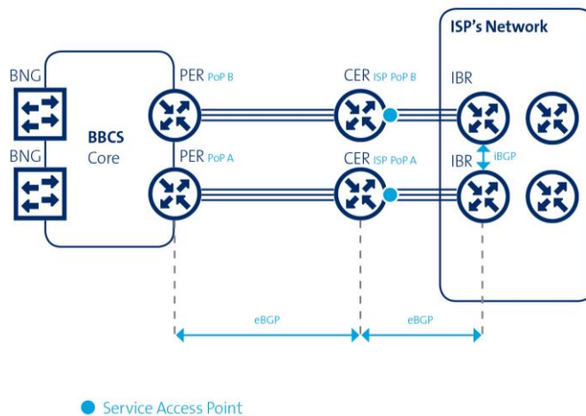
Abbildung 5: Übersicht BBCS Anbindung
