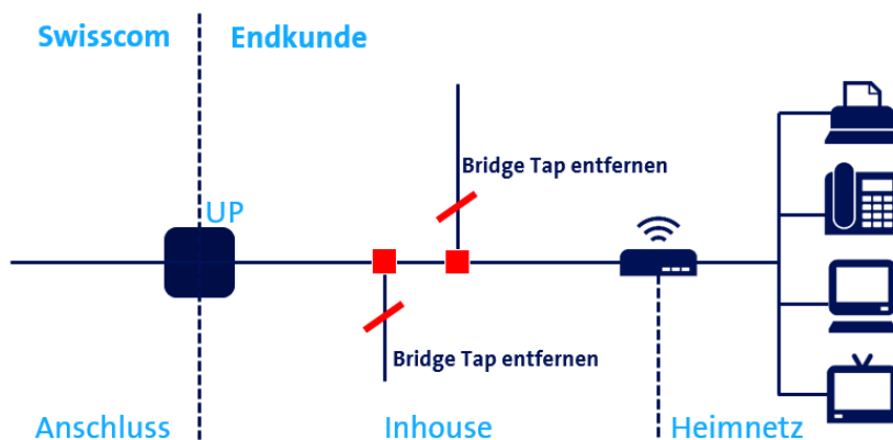
Abbildung 2: Installation bei Kupferleitungen
