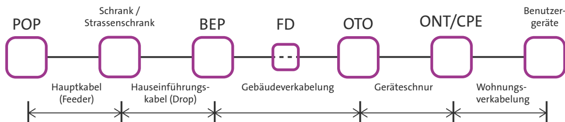
Abbildung 1: Referenzmodell BAKOM
