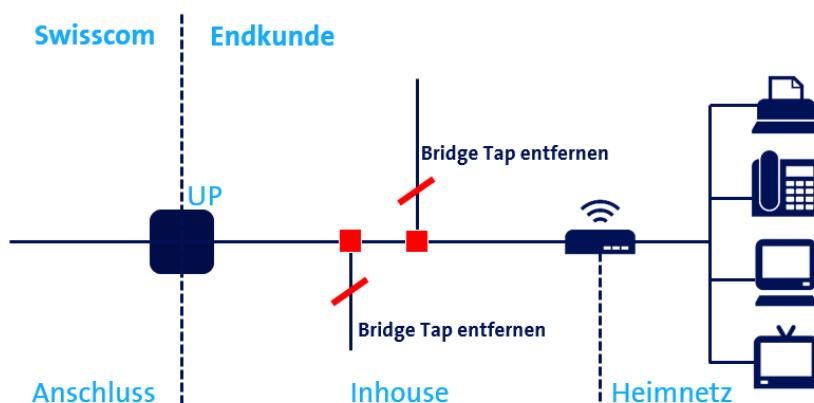
Abbildung 1: Installation bei Kupferleitungen
