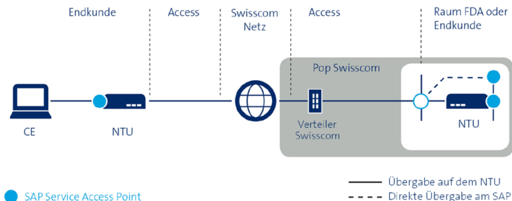
Illustration 2: Transfert du service CLS au sein du central de raccordement de Swisscom
