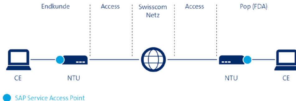
Illustration 1: Transfert du service CLS en dehors du central de raccordement Swisscom
