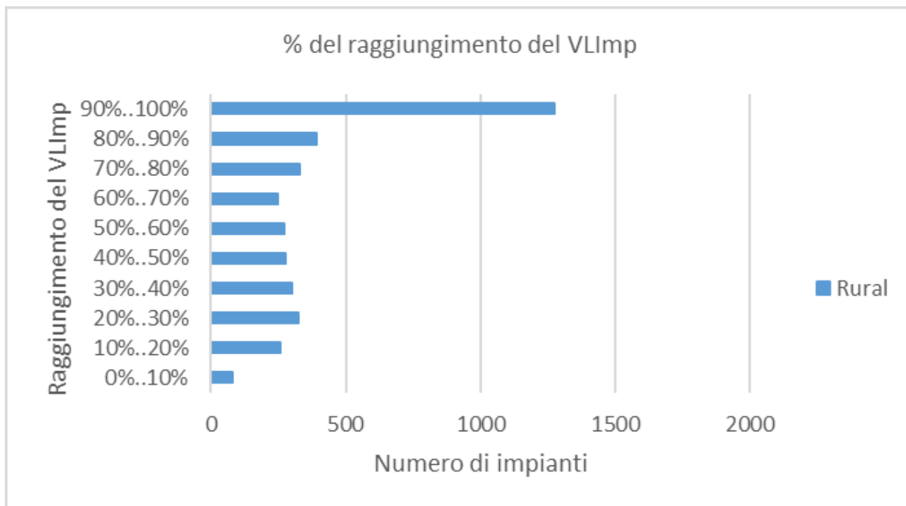
Figura 6: Raggiungimento del valore limite dell'impianto (aree rurali)
